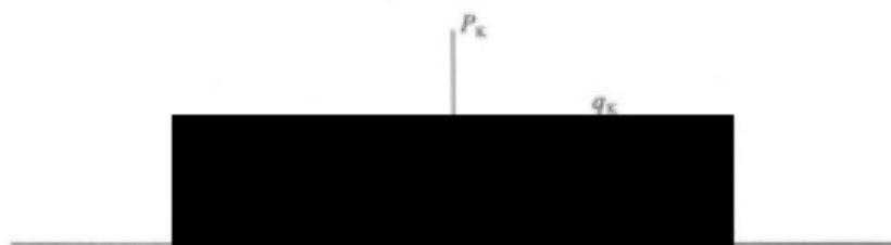
图 7.0.3 车道荷载
